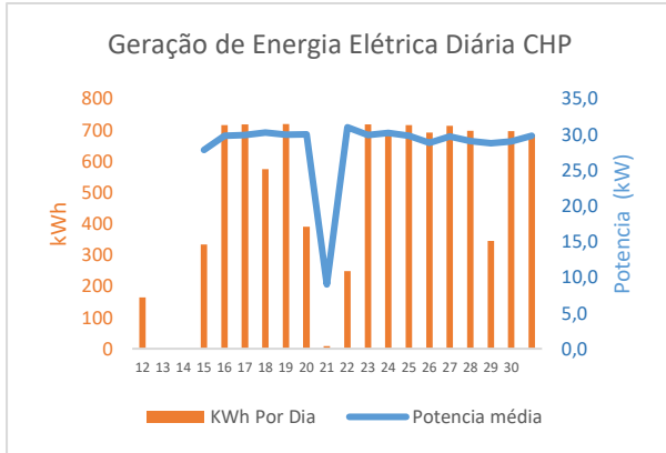
Figura 6 – Produção de energia do CHP
