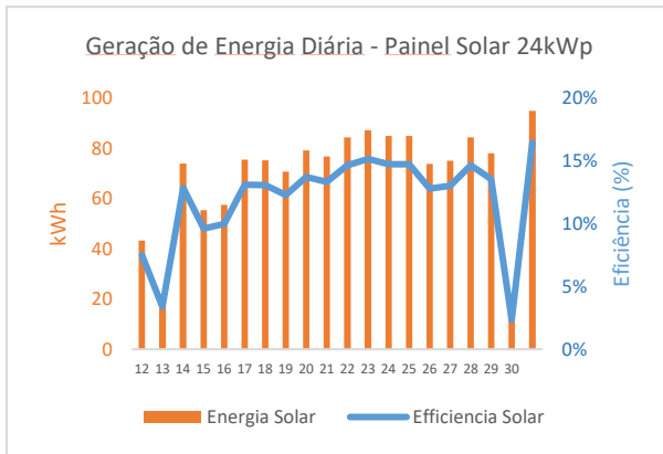
Figura 7 – Produção de energia solar
