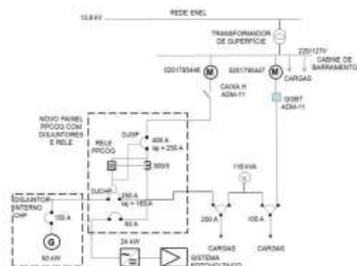
Figura 1 – Diagrama Unifilar Simplificado
