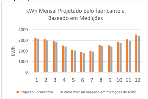
Figura 8 – Energia Pojetada vs. Medida
