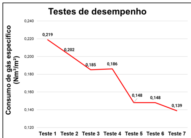
Figura 2. Consumo de gás em cada um dos testes realizados.
